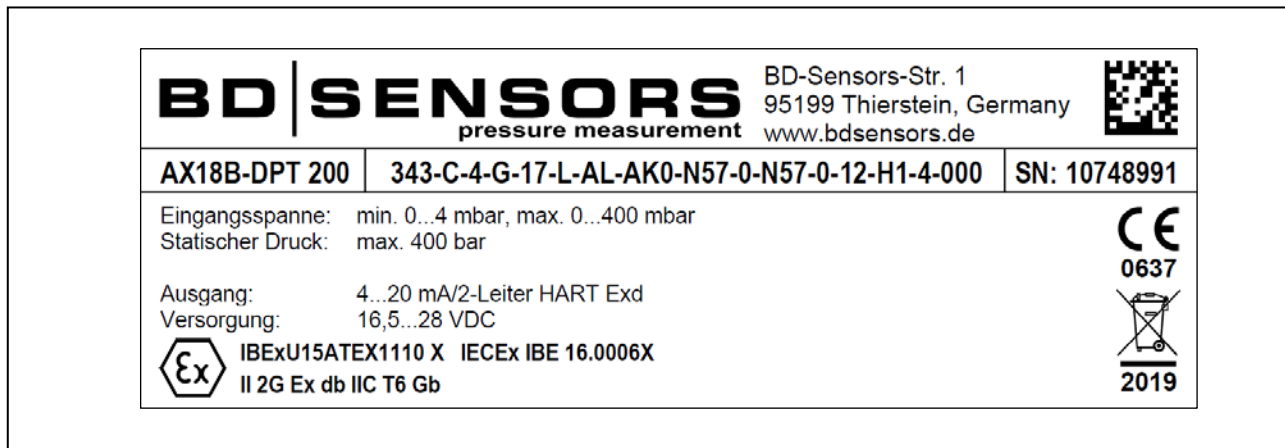
Abb. 2 Typenschildbeispiel Ex d
