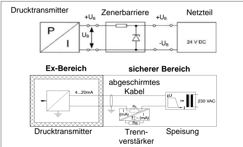
Abb. 3 Schaubild Beschaltung
