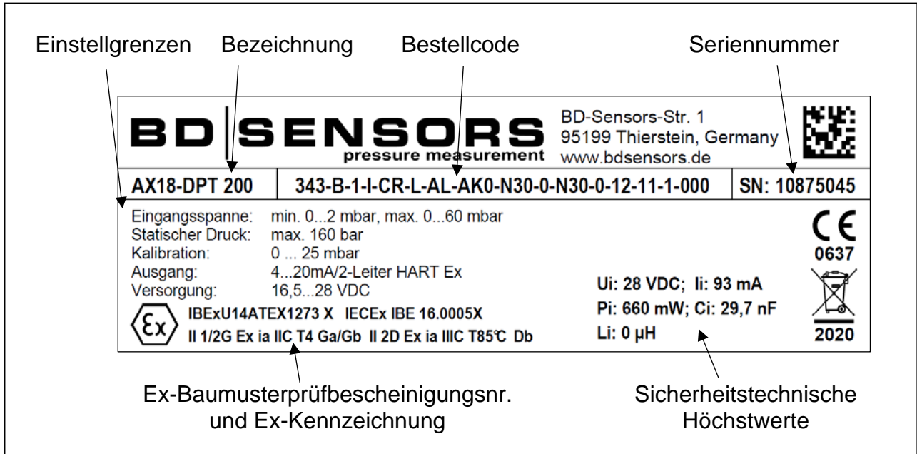
Abb. 1 Typenschildbeispiel Ex ia
